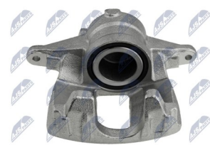
PINÇA TRAVAO FIAT FRT. ESQ. 52022042 BRAVO II 1.4 16V
