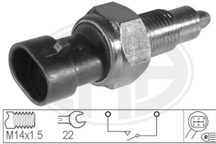
INTERRUPTOR LUZ M/A FIAT 46410523 PUNTO (188) = 40520+c
