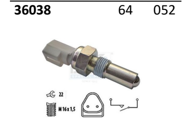
36038 64 052 INTERRUPTOR LUZ M/A FORD 2F 1029819 =40730 =330263
