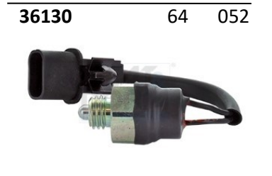
36130 64 052 INTERRUPTOR LUZ M/A HYUNDAI 938603D000 M14x2 EWCHY503
