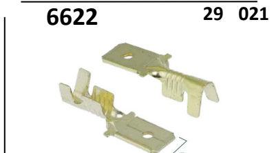
6622 29 021 TERMINAL MACHO 2.8mm 0.5-1mm
