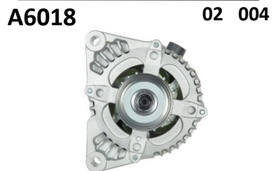
A6018 02 004 ALTERNADOR 12V 150A DENSO =113849 =CAL40195 =595545150
