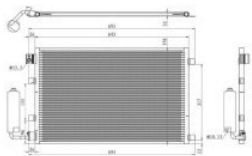
CONDENSADOR AC NISSAN =CCSNS027 667298 86SKV112
