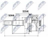
JOGO APOIO VEIO TRANSM. TO- 4234048030 4237049126 TRS. BLT.
