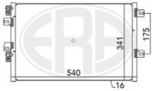
CONDENSADOR RENAULT =667073 =991079 CCSRE015
