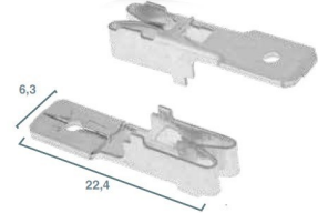
TERMINAL MACHO UNIV. F630
