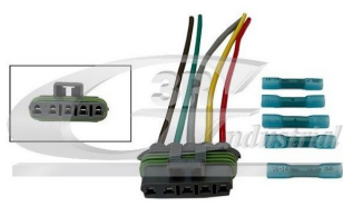
FICHA REP. MOTOR L/V PSA/FIAT 71774031 =25009 =53SKV235
