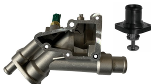
TERMOSTATO COMPLETO 1336S9 C4 C4 GRAND PICASSO I
