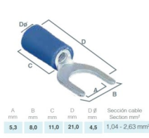
TERMINAL ISOLADO AZUL 1x2.5mm
