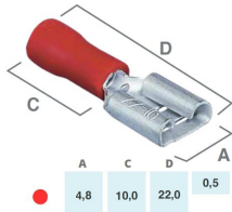
TERMINAL ISOLADO FEMEA P/FIO =1850300 =RO488
