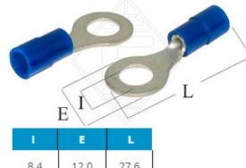
TERMINAL ISOLADO OLHAL AZUL P/FIO =1857250 =190039 =820
