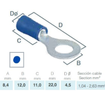
TERMINAL ISOLADO OLHAL AZUL P/FIO =1857250 =190039 =AZN084
