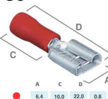
TERMINAL ISOLADO FEMEA VERME- =190022 =1851000 =RO638
