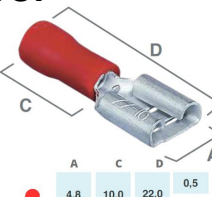
TERMINAL ISOLADO FEMEA P/FIO =1850500 =RO485
