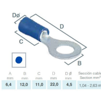
TERMINAL ISOLADO OLHAL AZUL =190034 =1857200 =AZN064
