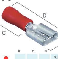
TERMINAL ISOLADO FEMEA VERME- 1901355866 =190049 =1850200
