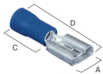
TERMINAL ISOLADO FÊMEA =1855000 =190020 =AZ638
