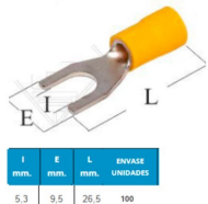
TERMINAL ISOLADO OLHAL P/FIO =1863150 =919
