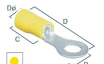
TERMINAL ISOLADO OLHAL AMARELO =190035 =1863200 =AMN064
