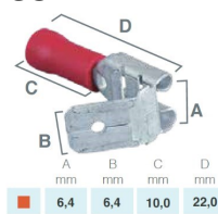
TERMINAL ISOLADO DUPLO 1901360820 =1852500 =RO6382
