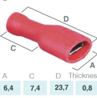
TERMINAL ISOLADO FEMEA VERME- P/FIO =190985 =1851500 =RO638F
