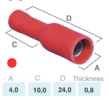
TERMINAL ISOLADO FEMEA VERME- =190017 =1864100 =RO395F
