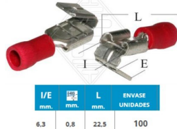
TERMINAL ISOLADO DUPLO 1901360821 =1862500 =838
