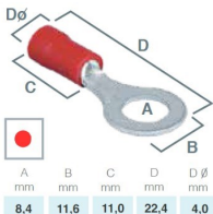
TERMINAL ISOLADO OLHAL =1853250 =192352 =RON084
