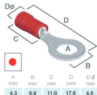
TERMINAL ISOLADO OLHAL =1853070 =190027
