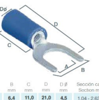
TERMINAL ISOLADO 4.3 1.4-2.63m
