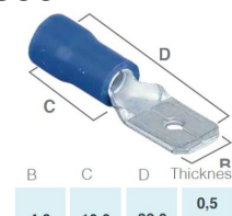
TERMINAL ISOLADO MACHO
