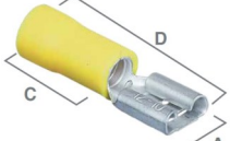
TERMINAL ISOLADO FÊMEA AMARELO P/FIO =190048 =1863000 =AM950C
