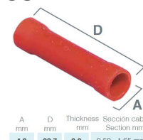
TERMINAL TODO ISOLADO VERMELHO =190028 =1868000 =RO170L
