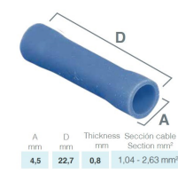
TERMINAL TODO ISOLADO AZUL =190001 =1868100 =AZN230L
