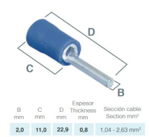
TERMINAL ISOLADO PONTA 1x2.5mm
