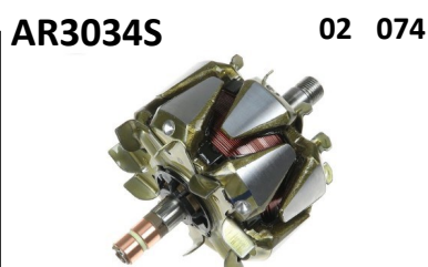
AR3034S 02 074 ROTOR ALT. 12V VALEO 593973/595403
