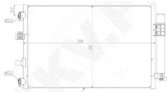
CONDENSADOR AC FORD 1703509 =667176 =CCSFR022
