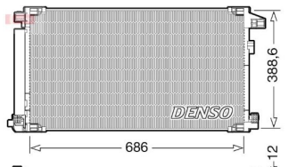
CONDENSADOR AC TOYOTA 8846010320 CCSTY035 350500
