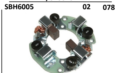
SUP. ESCOVAS M/A DENSO 0285105360 CBH40105AS
