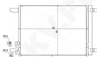
CONDENSADOR AC VAG 5Q0816411BC 86SKV227
