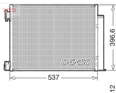
CONDENSADOR AC NISSAN 921005FA0A 86SKV241 090571050
