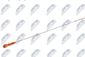
VARETA NIVEL OLEO PSA 655mm 1174F0 84214RG 8001081
